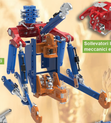
Tiranti Verticali meccanici e idraulici
